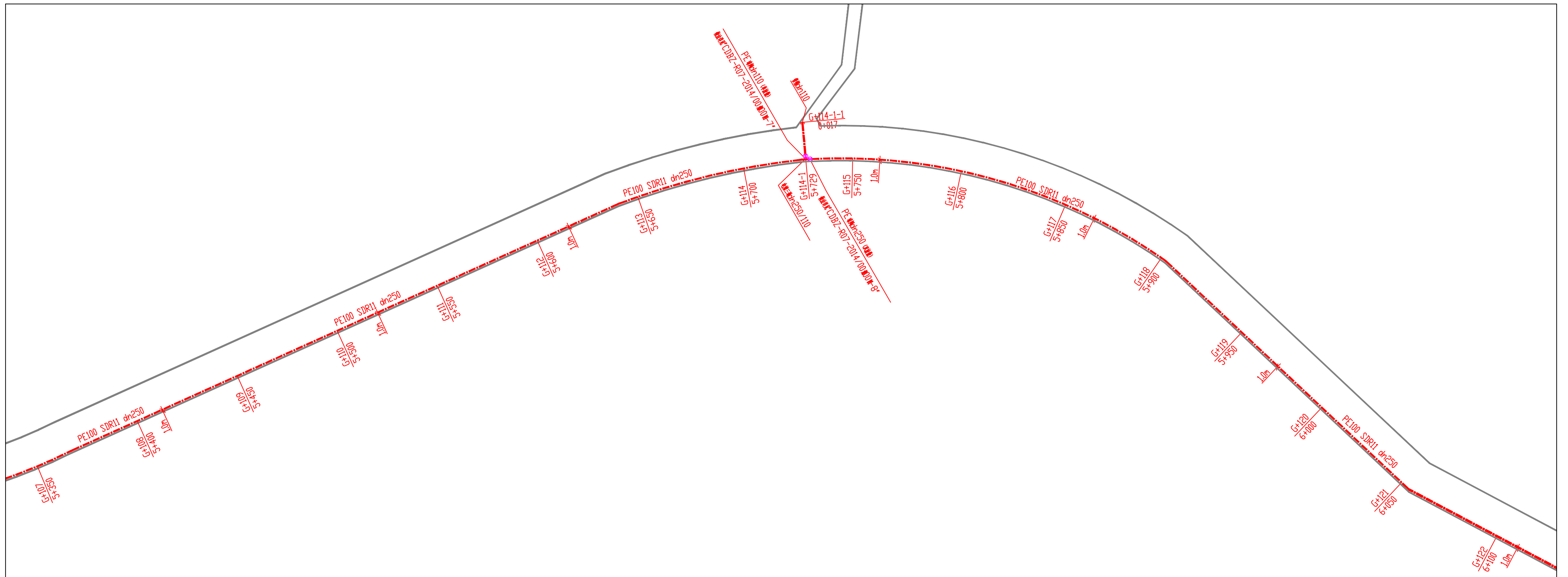
中压燃气管道平面布置图 (九) 1:1000
