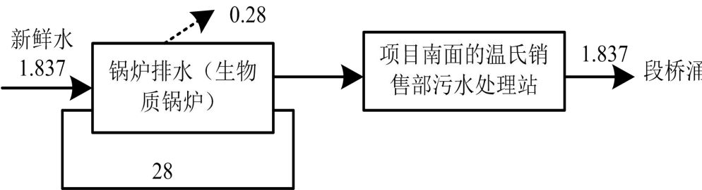
图 2-2 改扩建项目水平衡图（m³/d）
