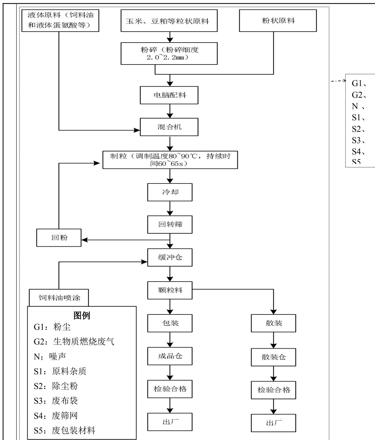
图2-4 本改扩建项目工艺流程及产污环节示意图
