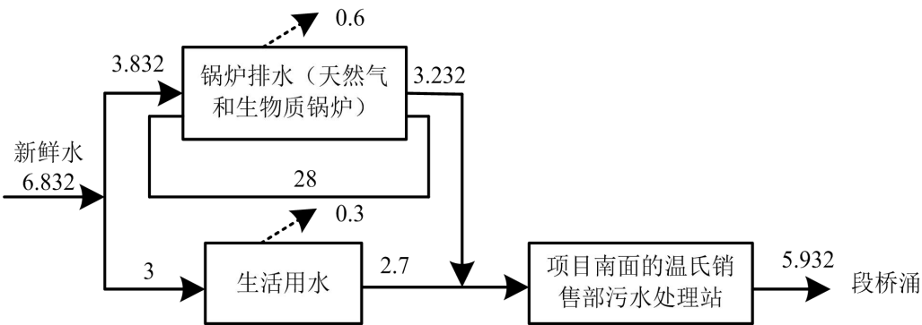
图 2-3 改扩建后项目总水平衡图（m³/d）
